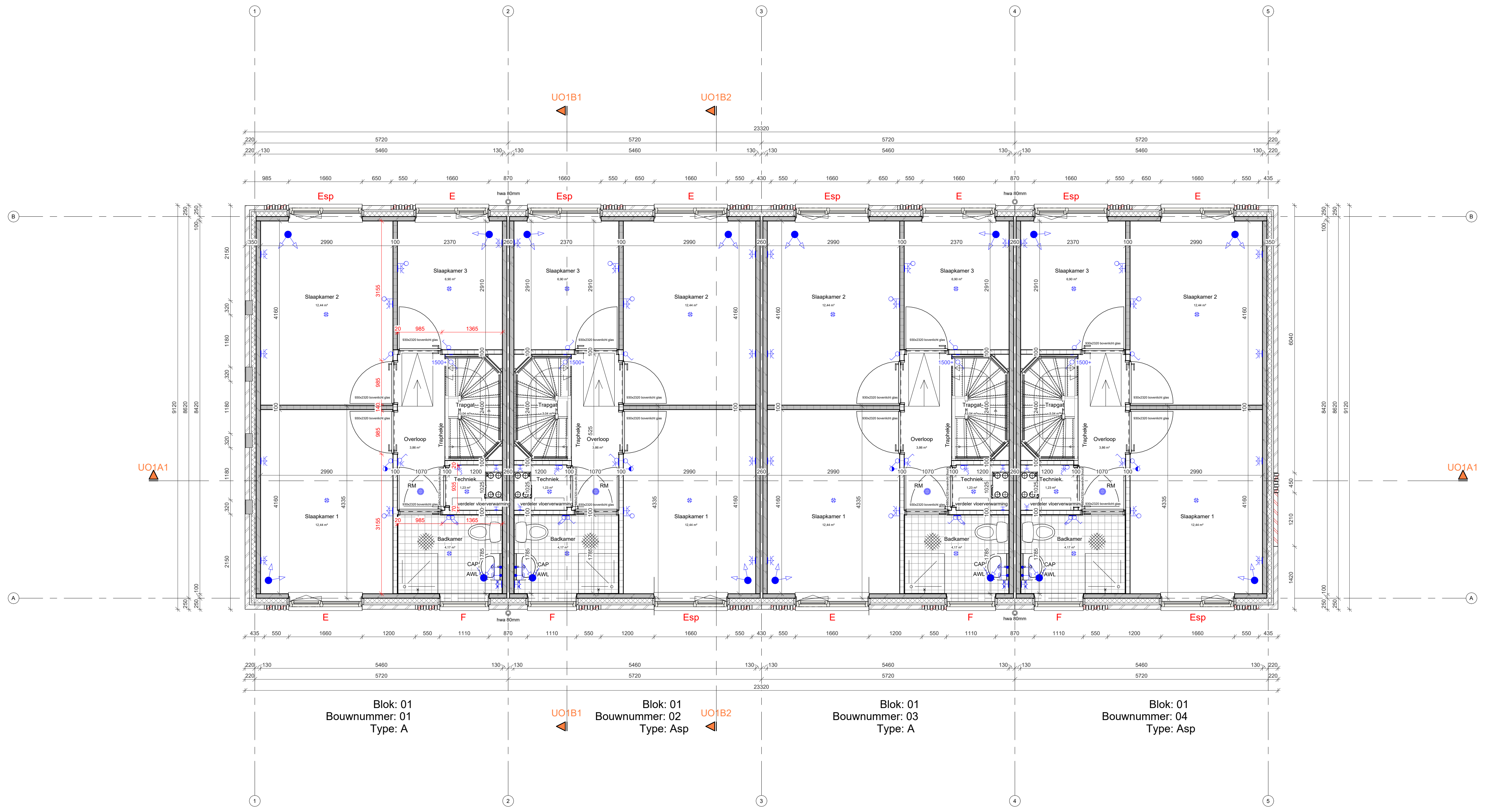
Eerste verdieping
