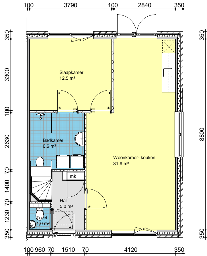
Begane grond
