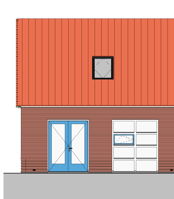
achtergevel
