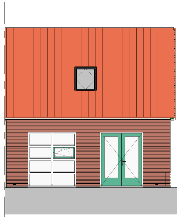
achtergevel
