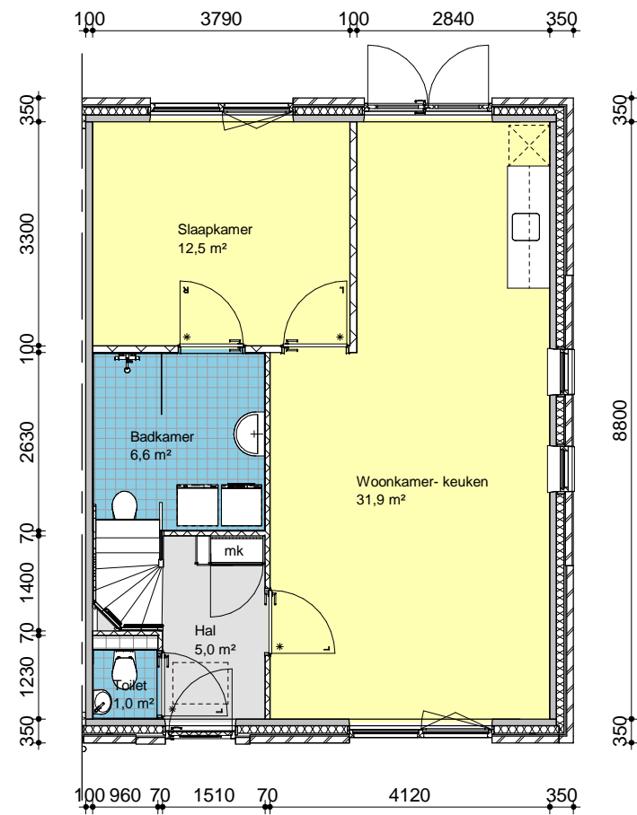
Begane grond
