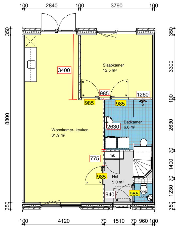
Begane grond
