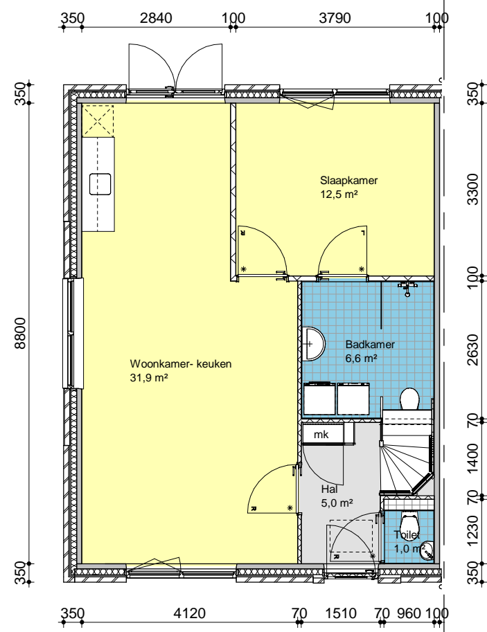
Begane grond
