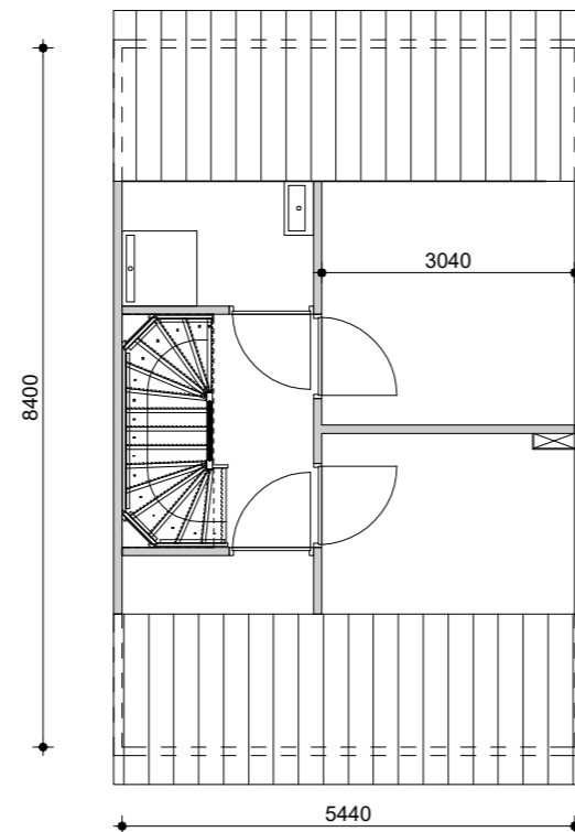
1e verdieping
