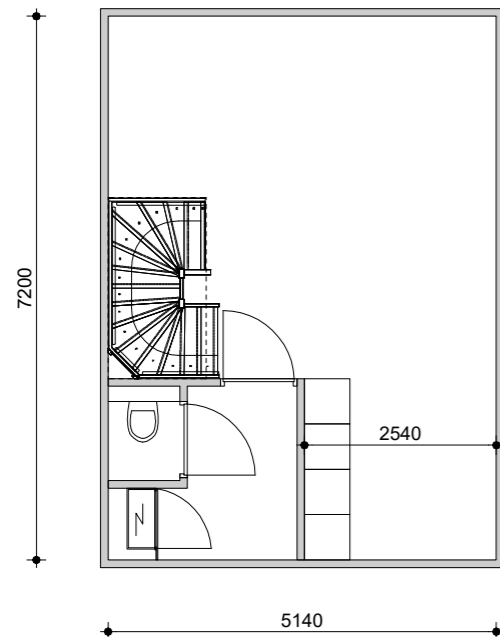
Begane grond
