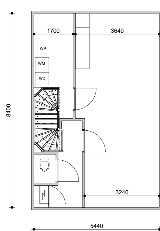
Begane grond
