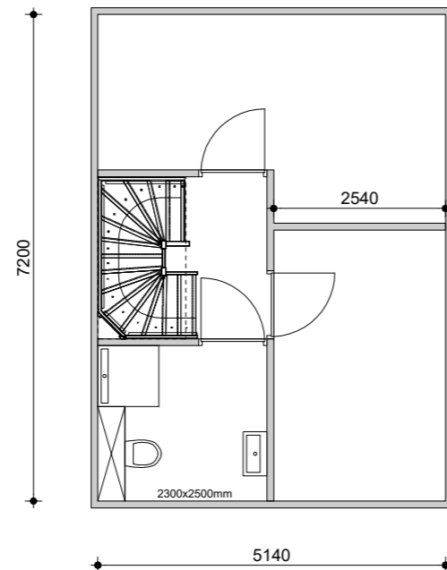
1e verdieping
